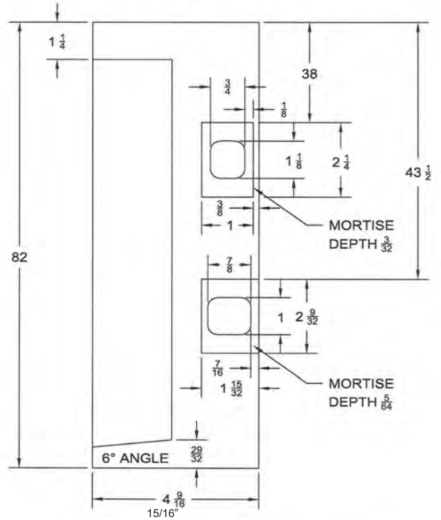
STRIKE JAMB 6/8
