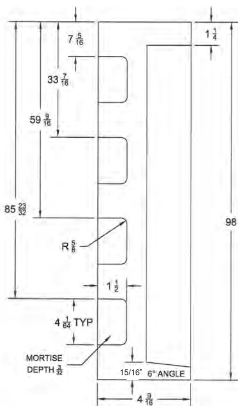
HINGE JAMB 8/0
