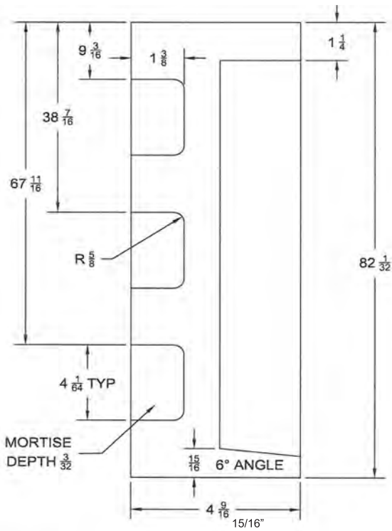
HINGE JAMB 6/8
